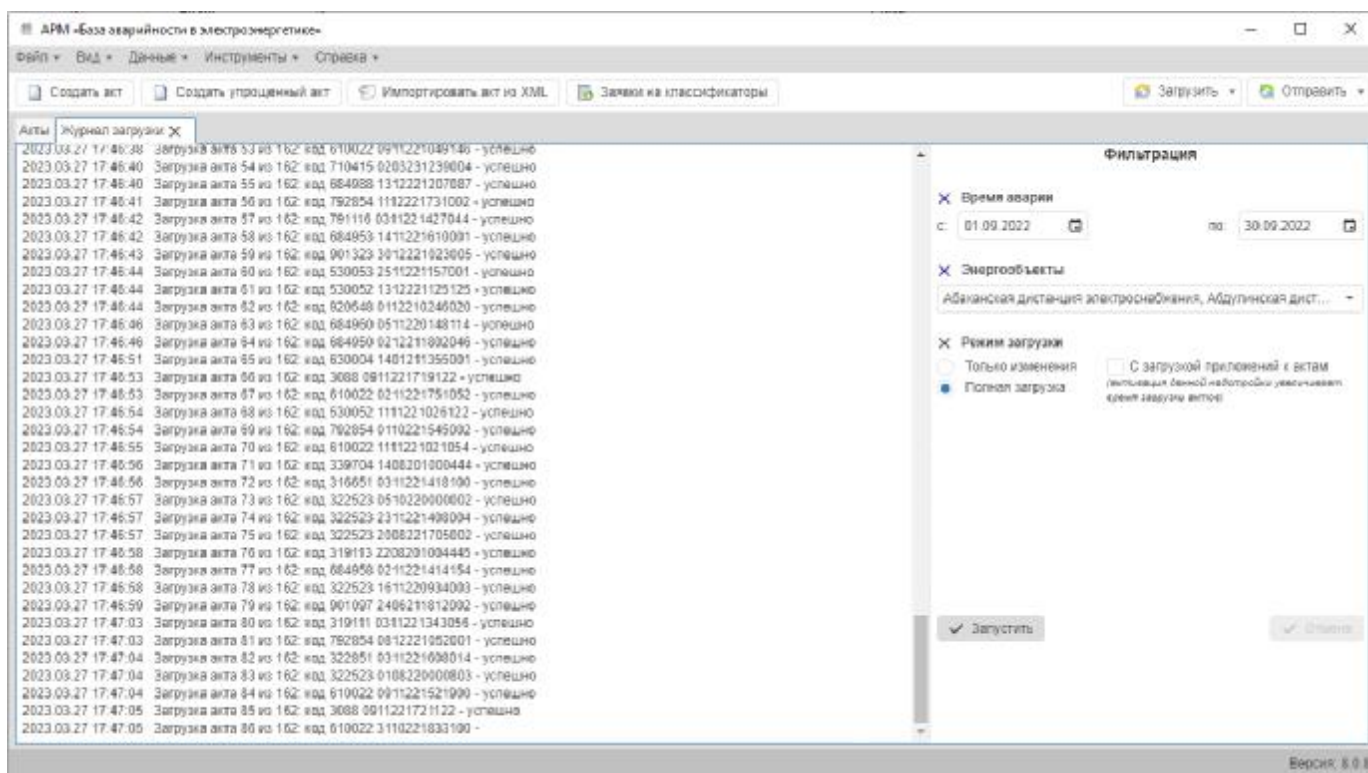
Рисунок 8.3 Окно отображения состояния загрузки актов
