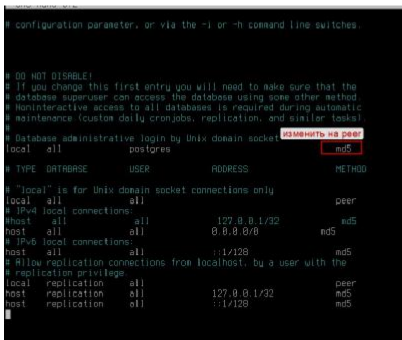
Рисунок 7.20 Изменение метода аутентификации
