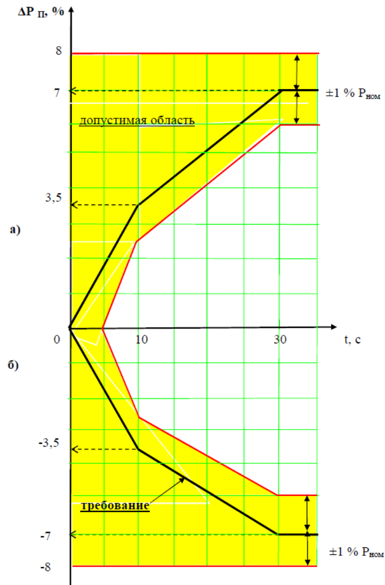
Рис.П.1. Допустимая область изменения первичной мощности гидроагрегата при \Delta P_{\text{П}} = \pm 7\% P_{\text{НОМ}} при скачкообразных снижении (а) и повышении (б)
