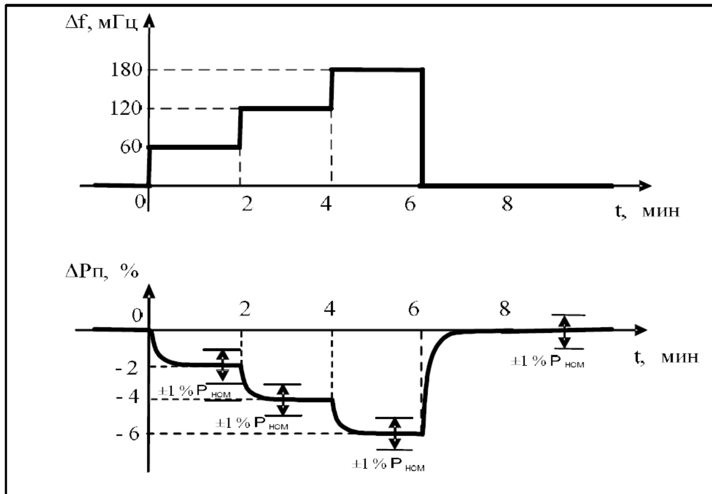
Рис.П.4. Имитация отклонений частоты в сторону увеличения и требуемые изменения первичной мощности гидроагрегата в следящем режиме Критерии оценки:
