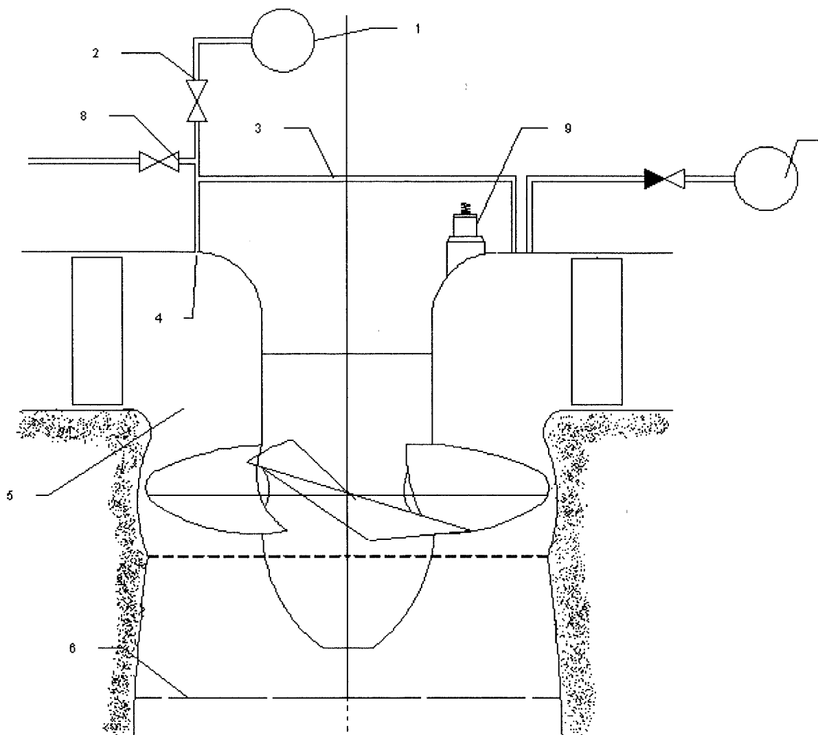
Рисунок В.1. Воздушная система отжатия воды из камеры рабочего колеса поворотно-лопастной гидротурбины: 1- Магистраль воздушной системы; 2- клапан пуска сжатого воздуха; 3-подводящий воздухопровод; 4-отверстия в крышке турбины; 5- камера рабочего колеса; 6- отжатый уровень воды; 7- устройство поддержания отжатого уровня; 8-клапан пуска атмосферного воздуха; 9- клапан срыва вакуума.
