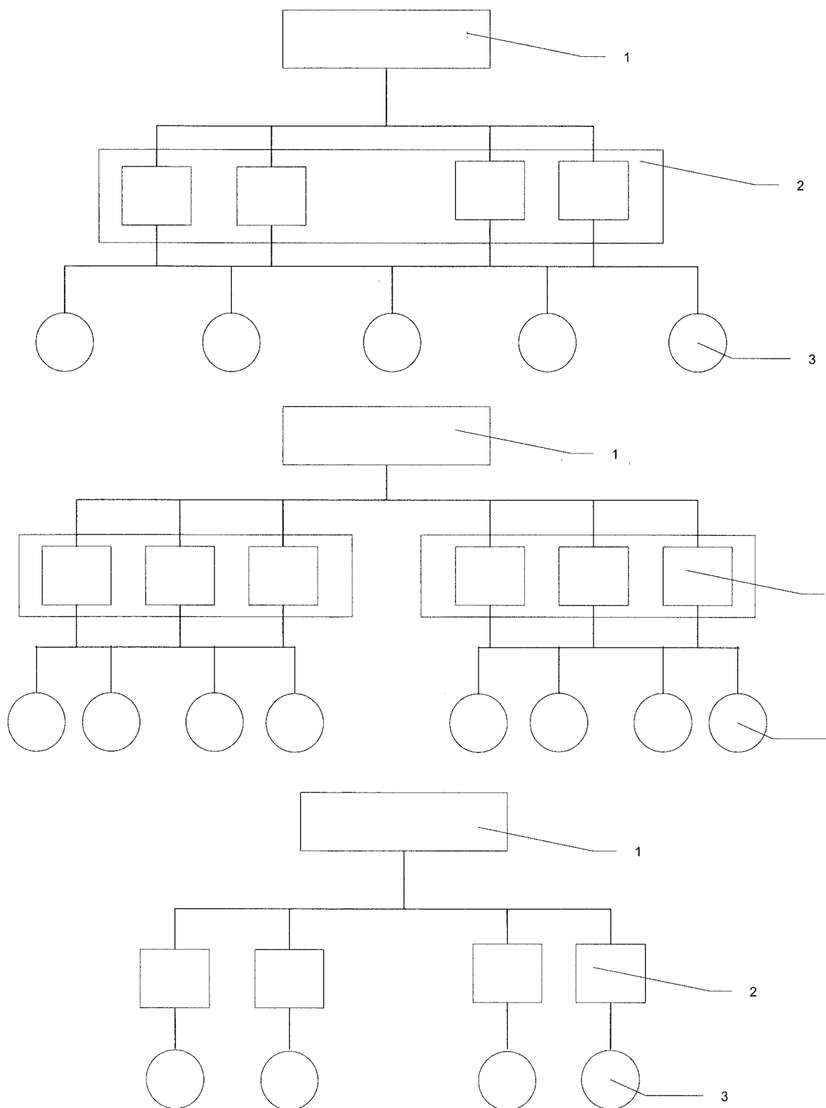
Рисунок В.5. Компоновка воздушной системы отжатия: объединенные (общестанционные)- верхняя схема, групповые (блочные)- средняя схема и индивидуальные (агрегатные)- нижняя схема. 1-компрессорная; 2-воздухосборник; 3-агрегат
