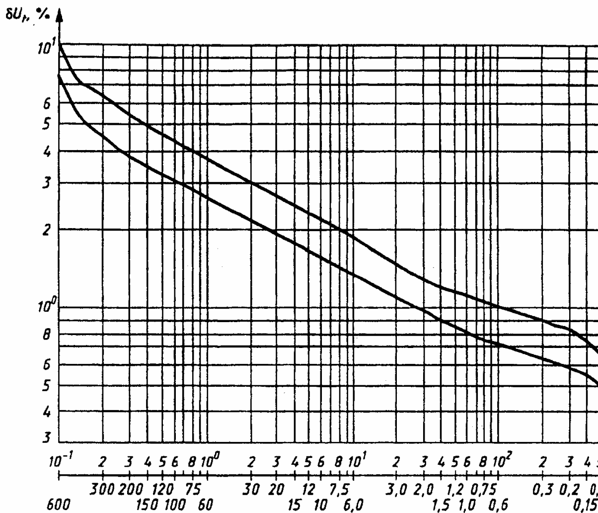
Рисунок 1 — Предельно допускаемые размахи изменений напряжения в зависимости от частоты повторения изменений напряжения за минуту для колебаний напряжения, имеющих форму меандра
