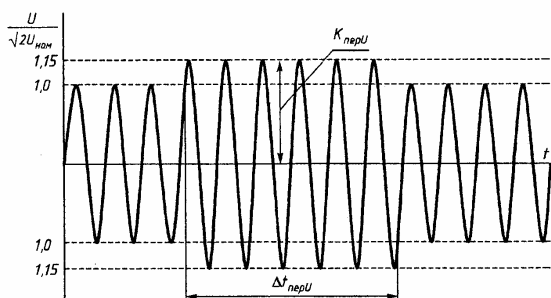
Рисунок Б.4 — Временное перенапряжение
