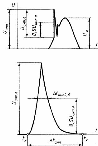
Рисунок Б.3 —Параметры импульсного напряжения
