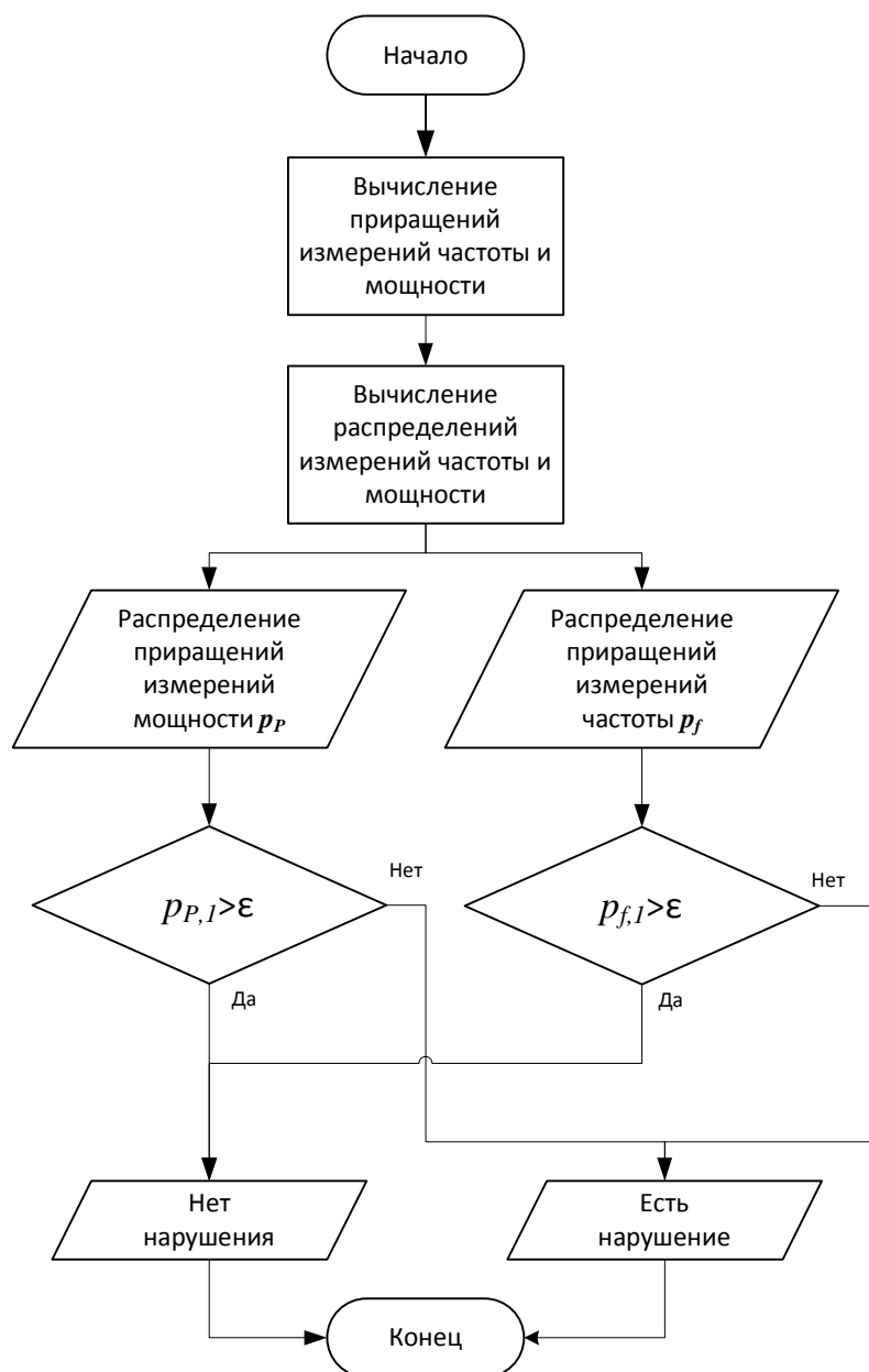
Рисунок 3. Блок-схема алгоритма "Несоответствие дискретности измерений требованиям"
