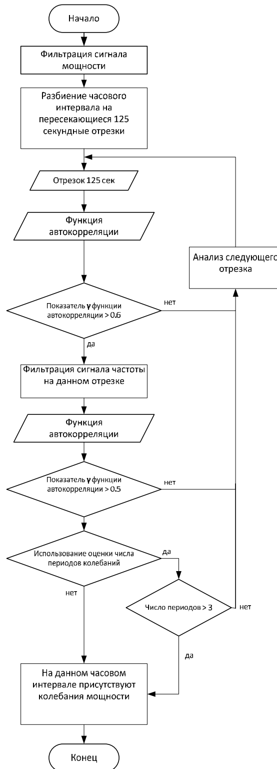
Рисунок 7. Блок-схема алгоритма "Наличие колебательного процесса"
