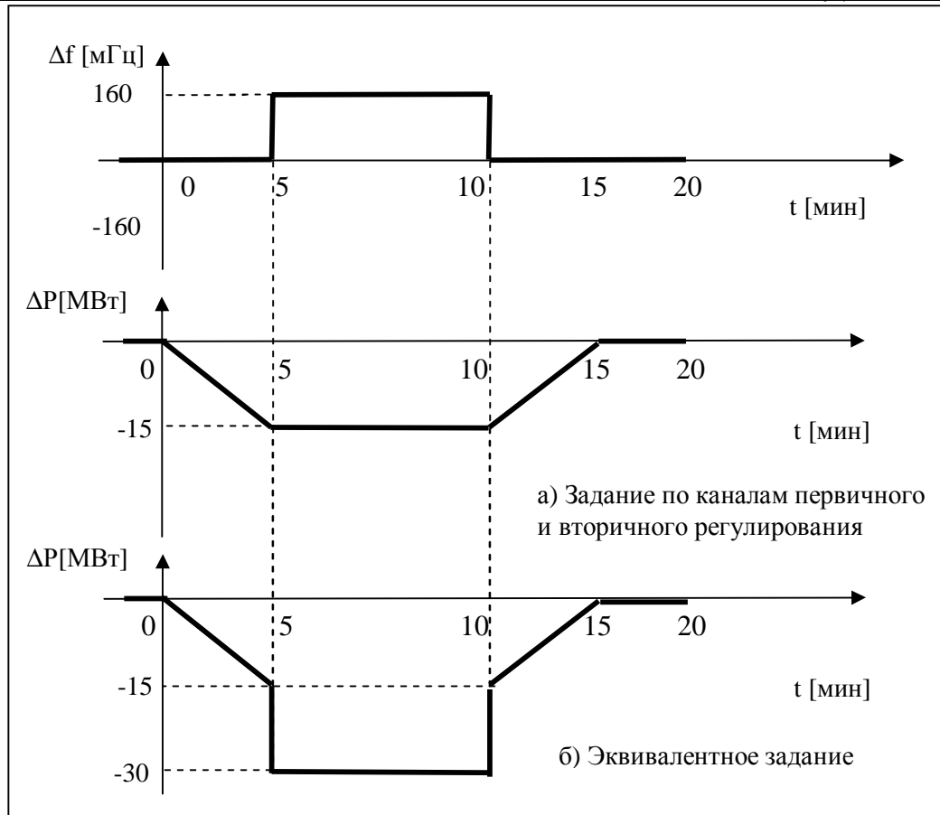
Рис. 8.7. Программа проверки энергоблоков в низу диапазона регулирования
