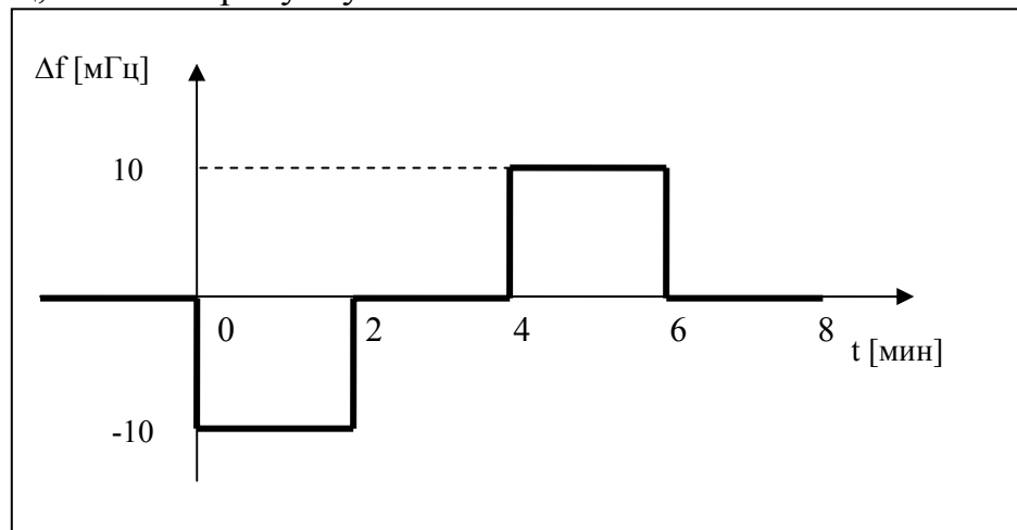
Рис. 8.1. Проверка нечувствительности первичных регуляторов.
