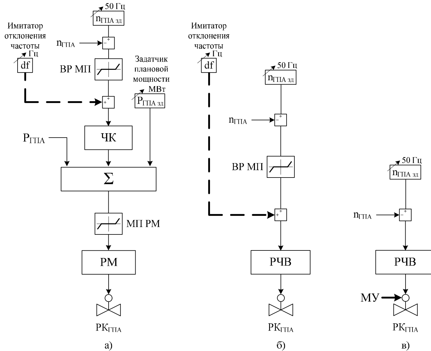
а) с РМ и ИОЧ; б) без РМ с ИОЧ; в) без РМ и ИОЧ Рисунок Г.8. Схема нанесения имитационных возмущений для ГПА
