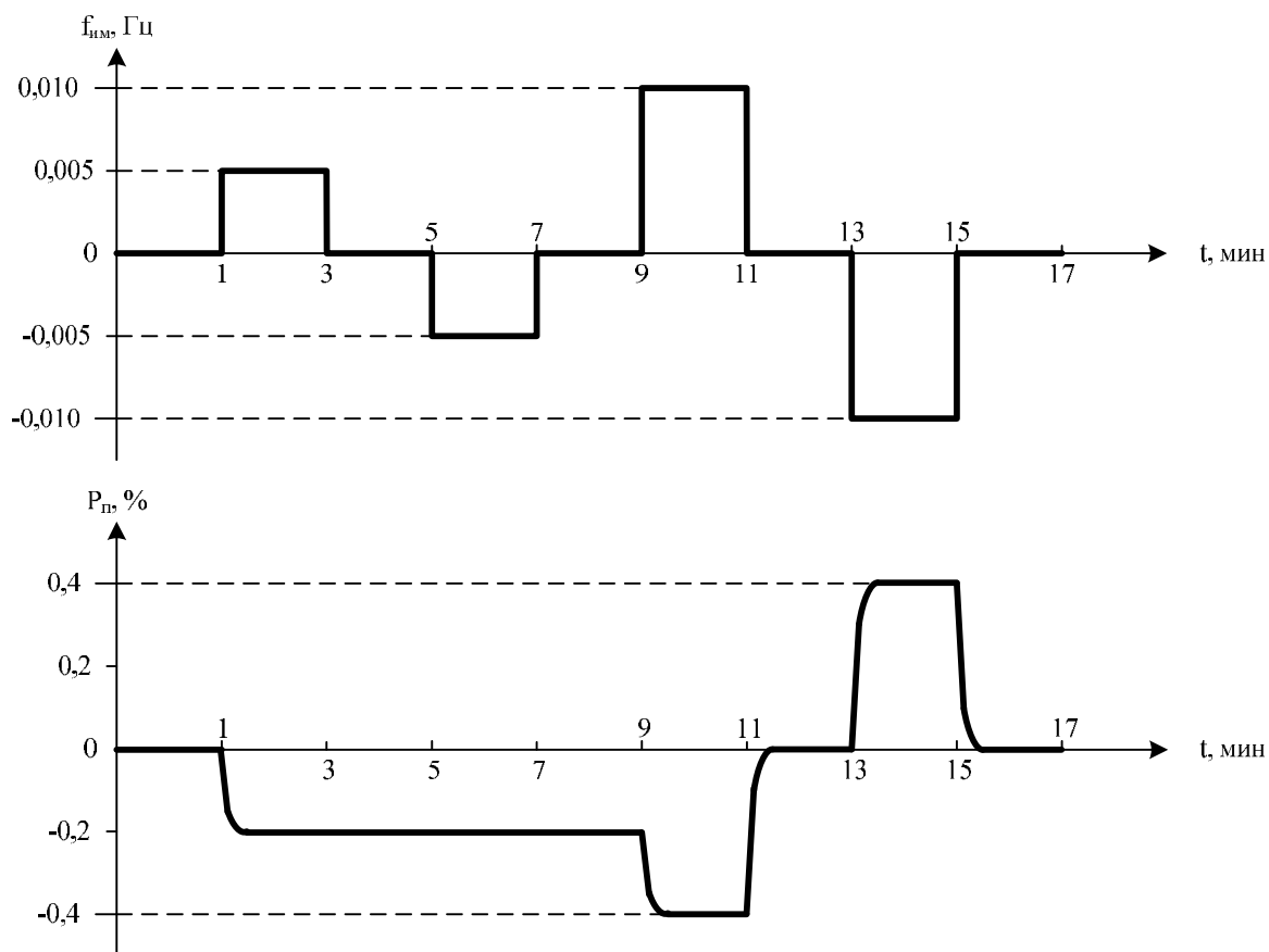
Рисунок 3. Последовательность нанесения и снятия имитационных отклонений частоты при оценке степени нечувствительности САРЧМ и один из вариантов соответствующего ему изменения мощности ( S = 5 \% , степень нечувствительности 10 мГц)
