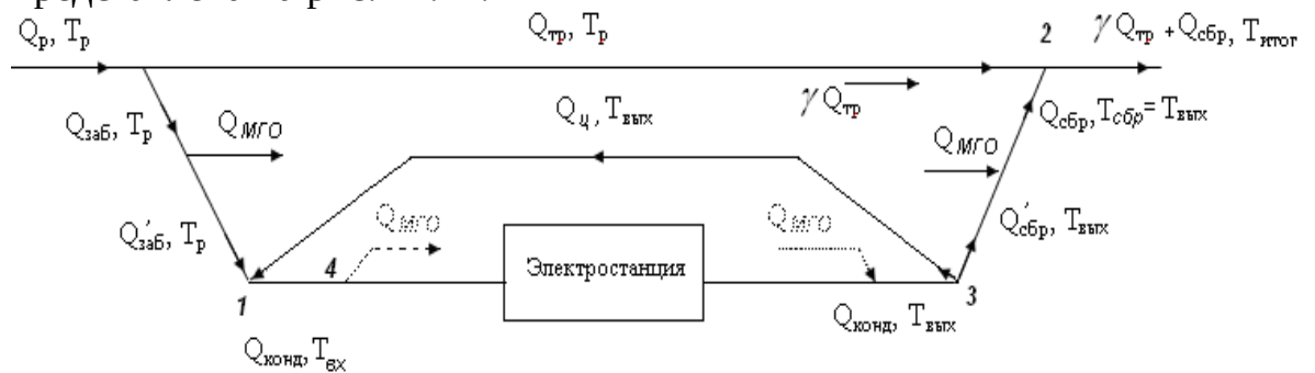
Рис. 11.11. Принципиальная схема технического водоснабжения
