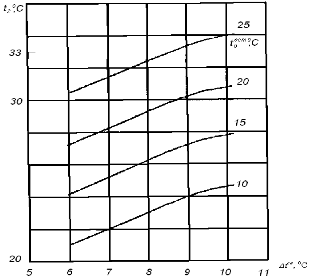
Рис. 11.8. Примерный вид зависимости t_2 = f(t_8^{ecm}; t^{cs})
