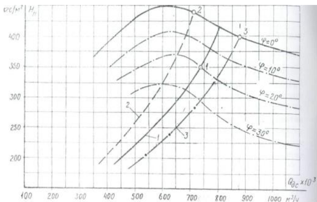
Рис. 14.1. Ограничение паропроизводительности котла из-за нехватки тяги: 1 – расчетная характеристика газового тракта; 2 – характеристика газового тракта при загрязнениях конвективной шахты; 3 – характеристика газового тракта при увеличенных присосах холодного воздуха.
