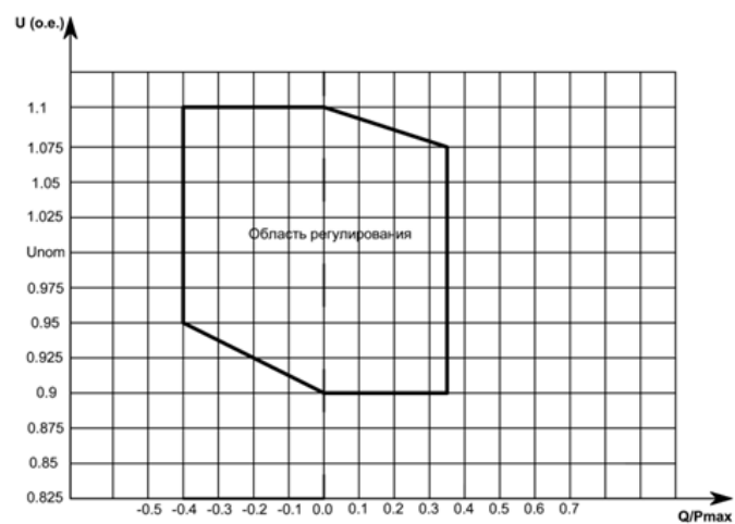
Рис. П1.2. Зависимость регулировочного диапазона по реактивной мощности ВИЭ от фактического напряжения в точке подключения к сети. (U-Q диаграмма).
