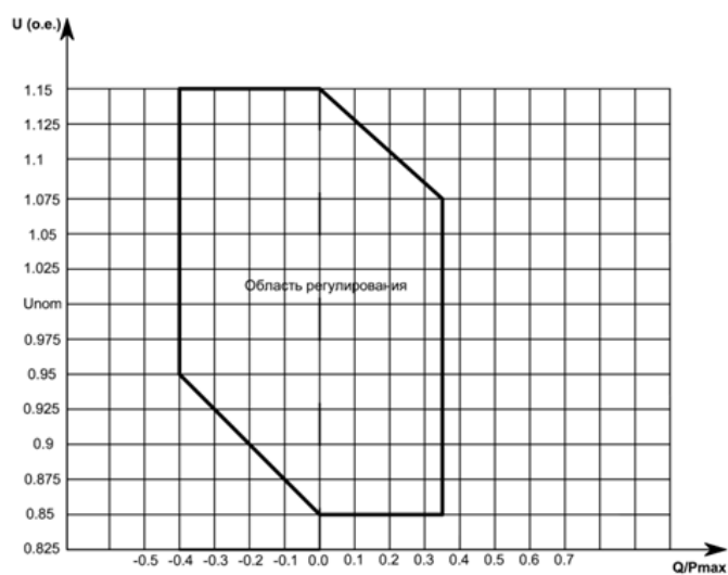
Рис. П1.2. Зависимость регулировочного диапазона по реактивной мощности ВИЭ от фактического напряжения в точке подключения к сети. (U-Q диаграмма).
