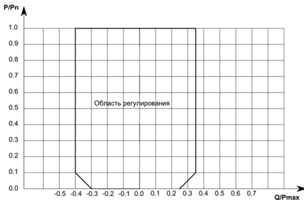
Рис. П1.1. Зависимость регулировочного диапазона по реактивной мощности ВИЭ от её фактической генерации активной мощности (P-Q диаграмма).
