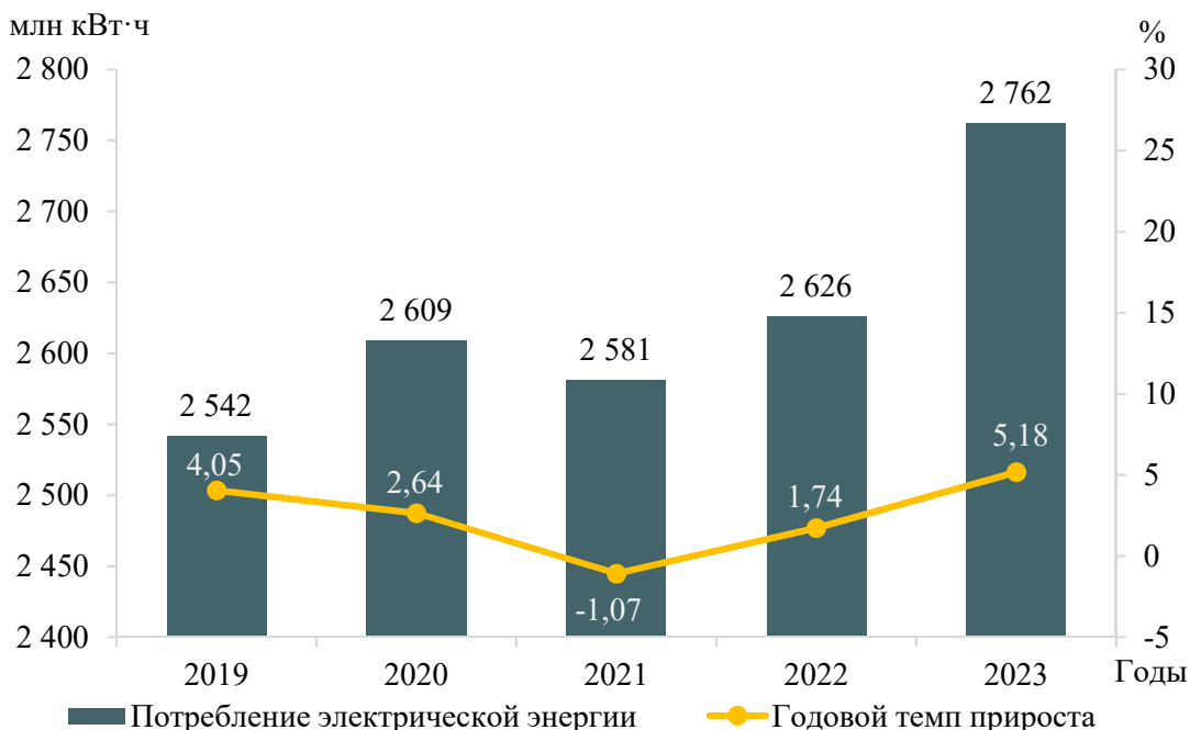
Рисунок 1 – Потребление электрической энергии электроэнергетической системы Сахалинской области и годовые темпы прироста
