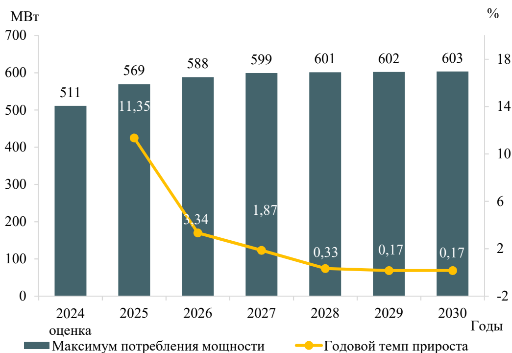
Рисунок 4 – Прогноз максимума потребления мощности электроэнергетической системы Сахалинской области и годовые темпы прироста
