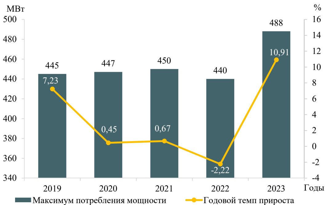
Рисунок 2 – Максимум потребления мощности электроэнергетической системы Сахалинской области и годовые темпы прироста
