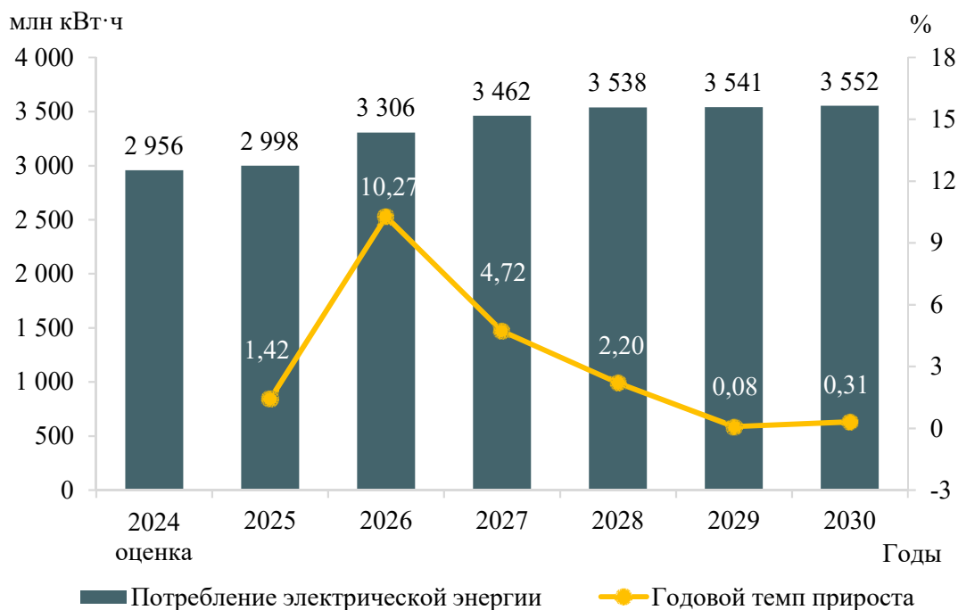
Рисунок 3 – Прогноз потребления электрической энергии электроэнергетической системы Сахалинской области и годовые темпы прироста
