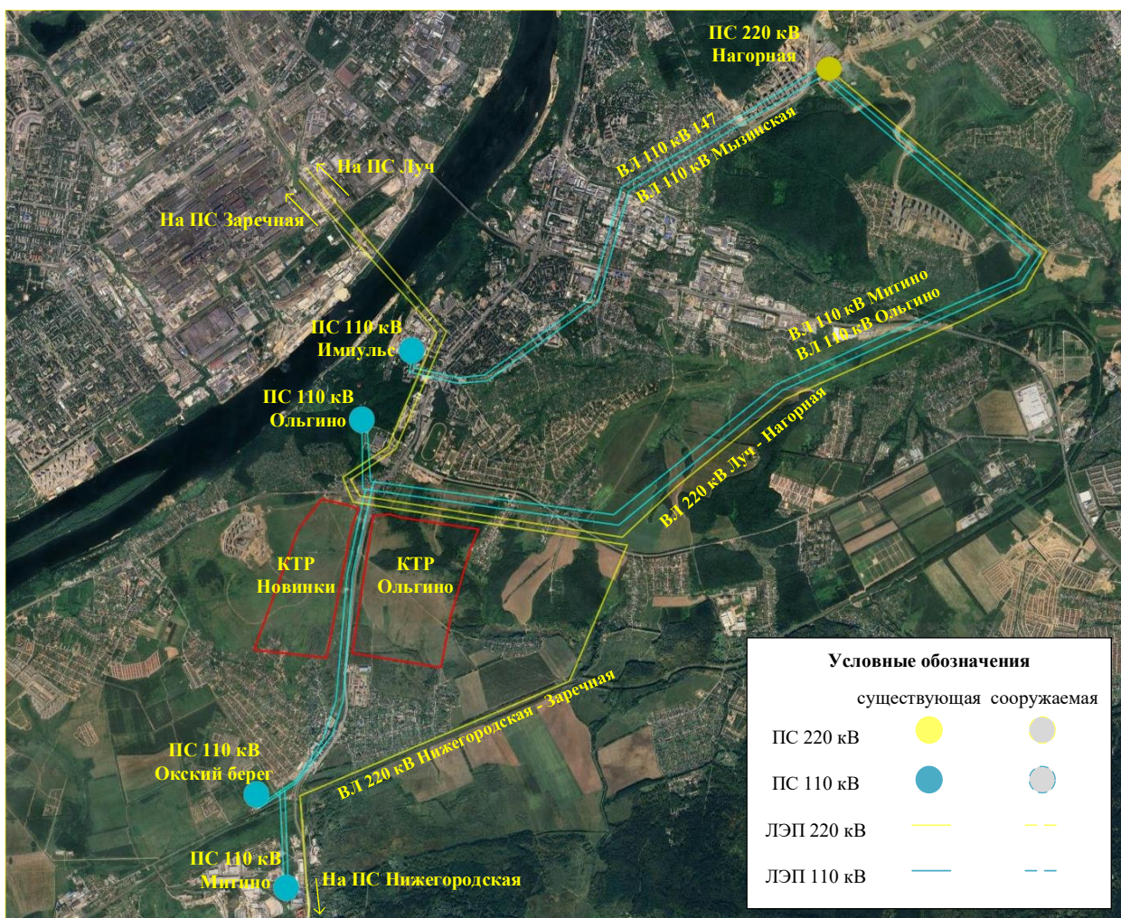
Рисунок 5 – Карта-схема электрических сетей района размещения потребителей КРТ Новинки, КРТ Ольгино
