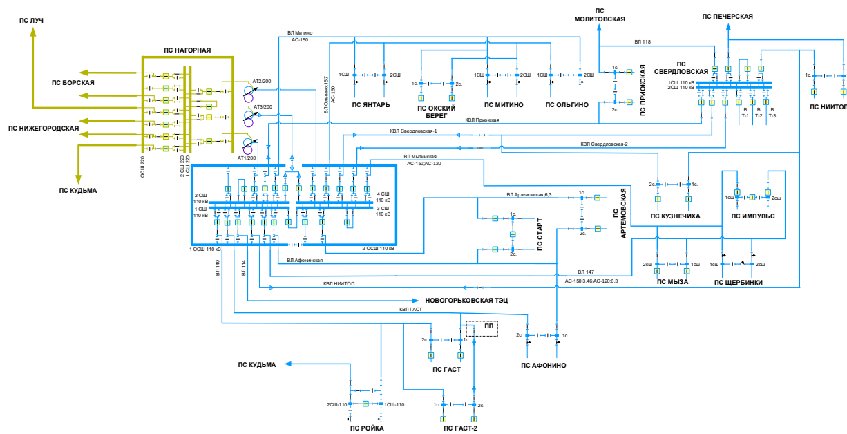
Рисунок 6 – Принципиальная схема электрической сети района размещения потребителей КРТ Новинки, КРТ Ольгино
