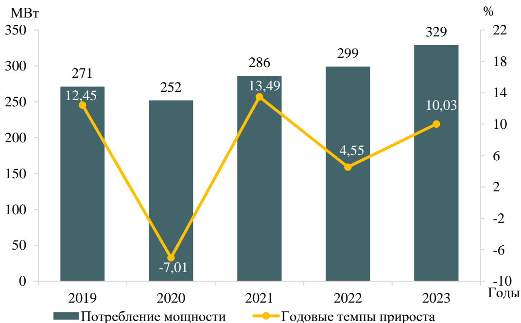
Рисунок 2 – Потребление мощности Еврейской автономной области и годовые темпы
