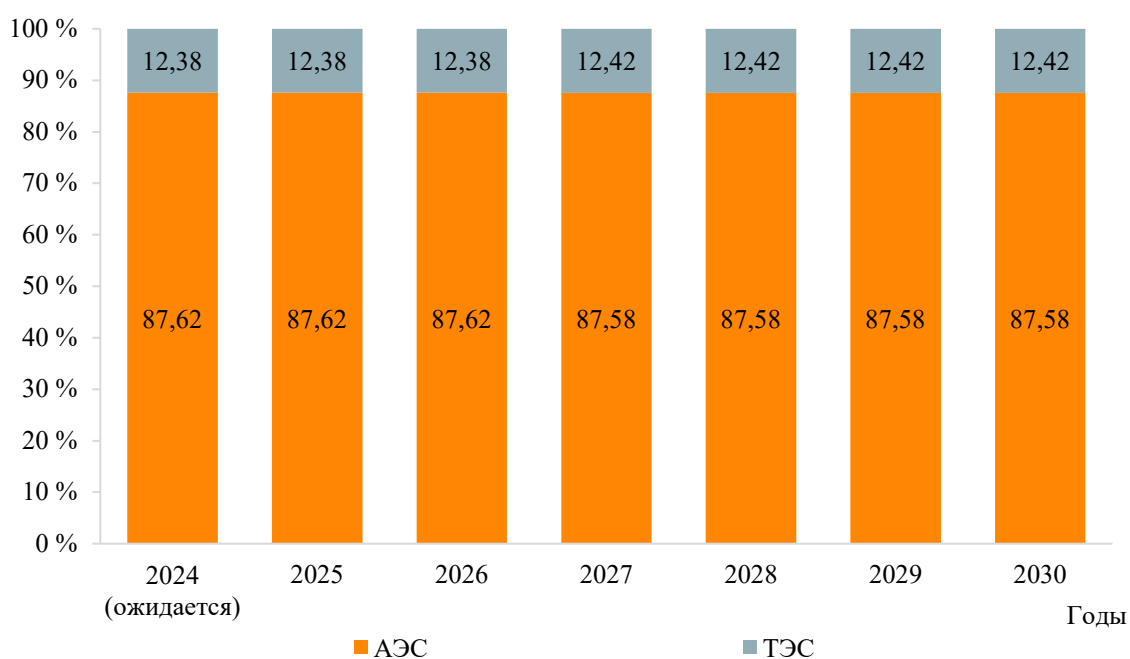
Рисунок 10 – Структура установленной мощности электростанций энергосистемы Воронежской области
