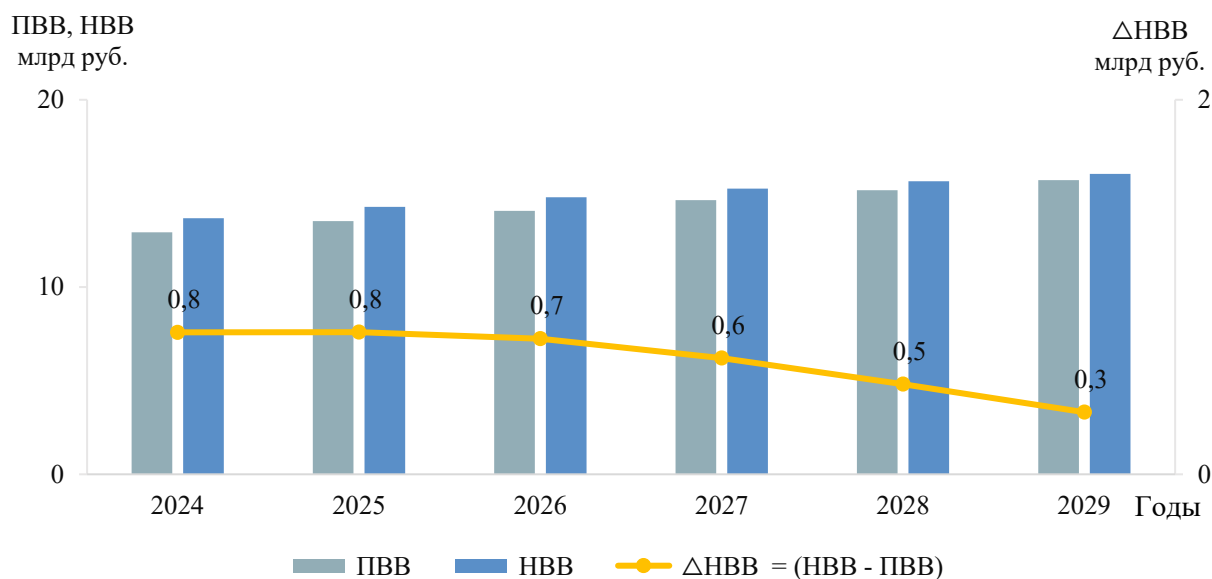
Рисунок 7 – Результаты оценки достаточности выручки, получаемой ТСО Ярославской области при существующих механизмах тарифного регулирования, для реализации планируемого состава технических решений, предлагаемых к включению в схему и программу развития электроэнергетических систем России (Базовый сценарий)
