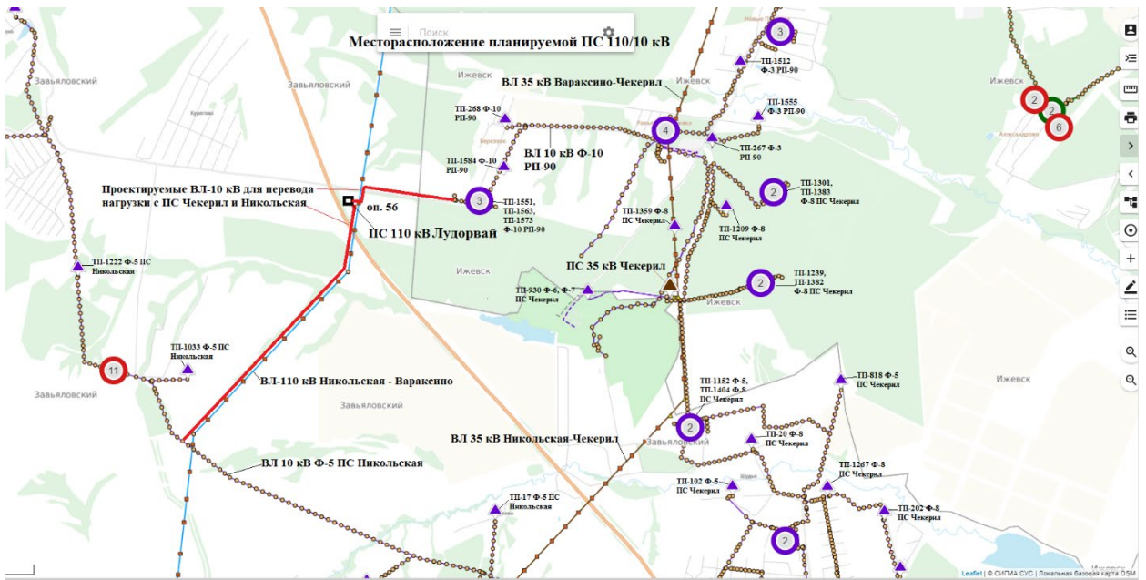
Рисунок 3 – Схема расположения новой ПС 110 кВ Лудорвай
