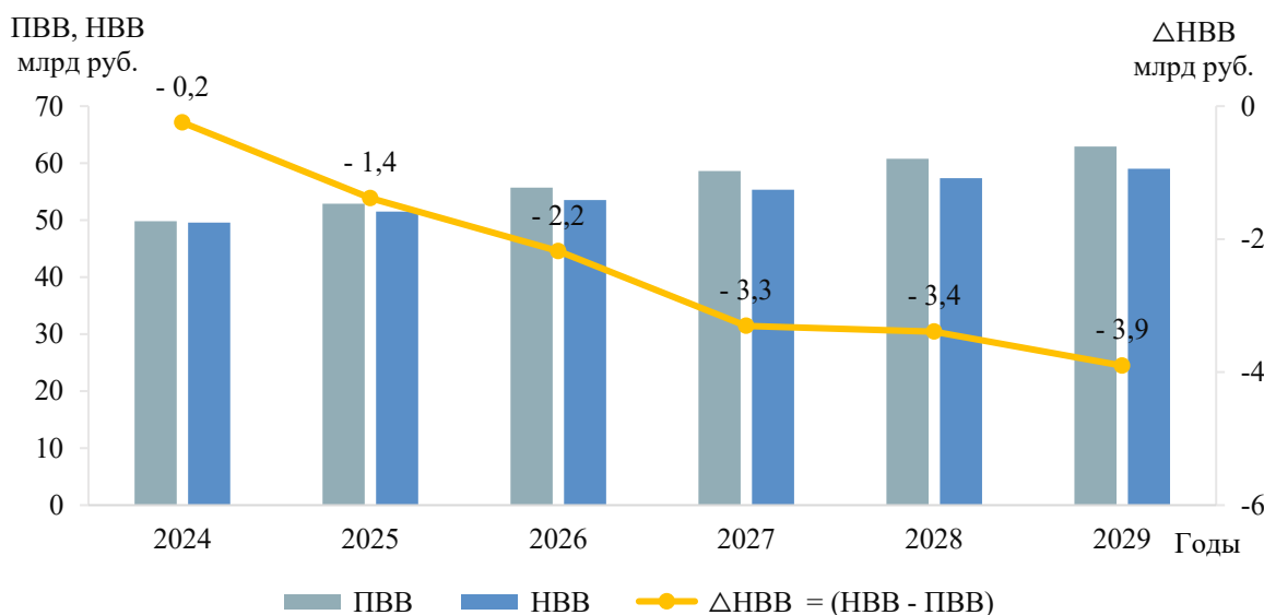
Рисунок 10 – Результаты оценки достаточности выручки, получаемой ТСО Свердловской области при существующих механизмах тарифного регулирования, для реализации планируемого состава технических решений, предлагаемых к включению в схему и программу развития электроэнергетических систем России (Базовый сценарий)
