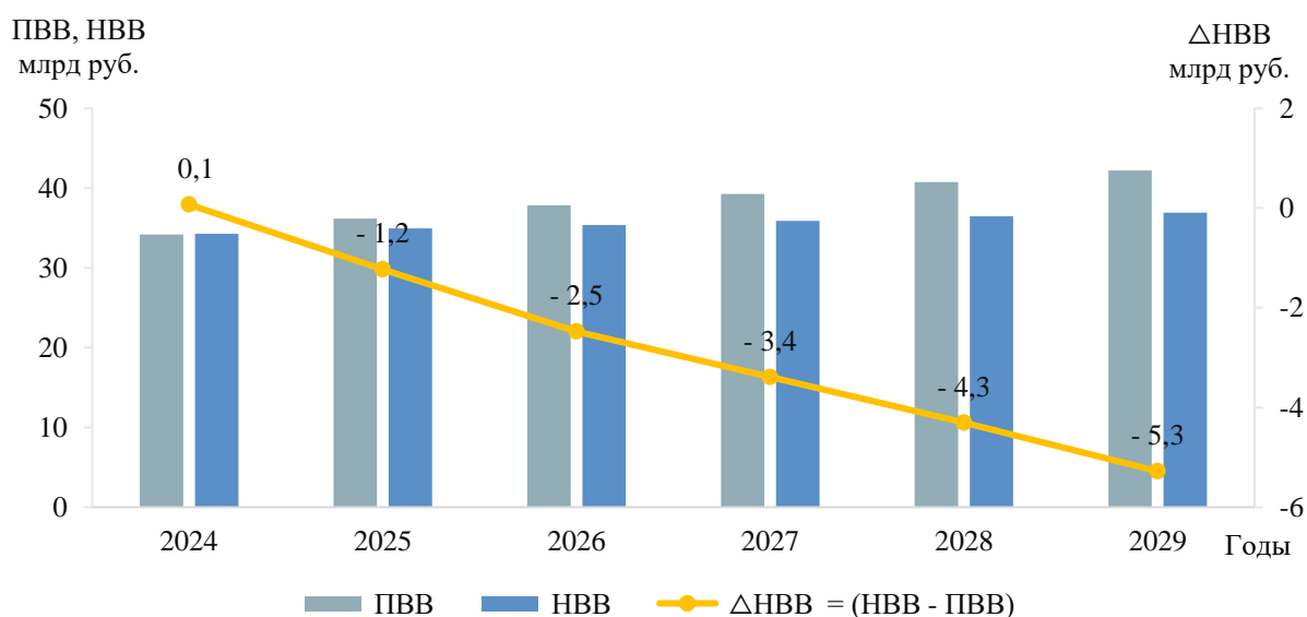
Рисунок 8 – Результаты оценки достаточности выручки, получаемой ТСО Республики Татарстан при существующих механизмах тарифного регулирования, для реализации планируемого состава технических решений, предлагаемых к включению в схему и программу развития электроэнергетических систем России (Базовый сценарий)
