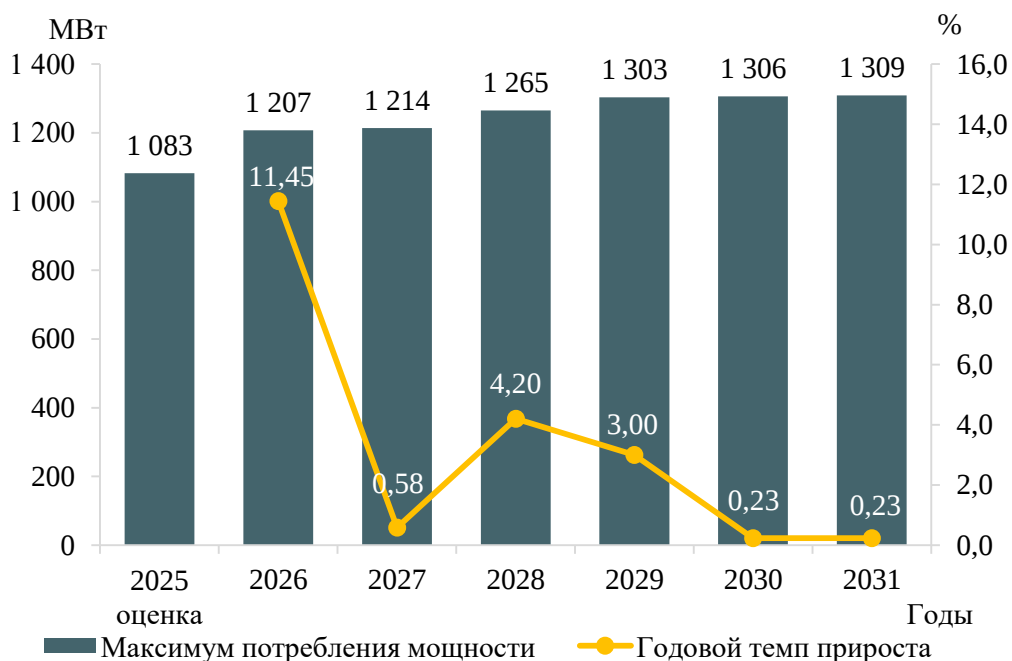
Рисунок 7 – Прогноз максимума потребления мощности электроэнергетической системы Таймырского Долгано-Ненецкого муниципального района, Туруханского района и городского округа г. Норильск Красноярского края и годовые темпы прироста
