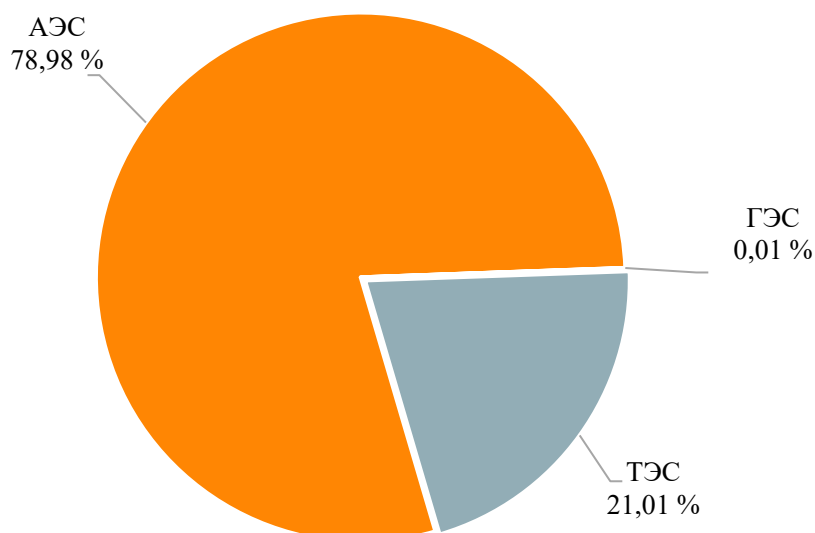
Рисунок 2 – Структура производства электрической энергии электростанций энергосистемы Тверской области в 2024 году
