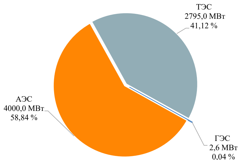
Рисунок 1 – Структура установленной мощности электростанций энергосистемы Тверской области по состоянию на 01.01.2025
