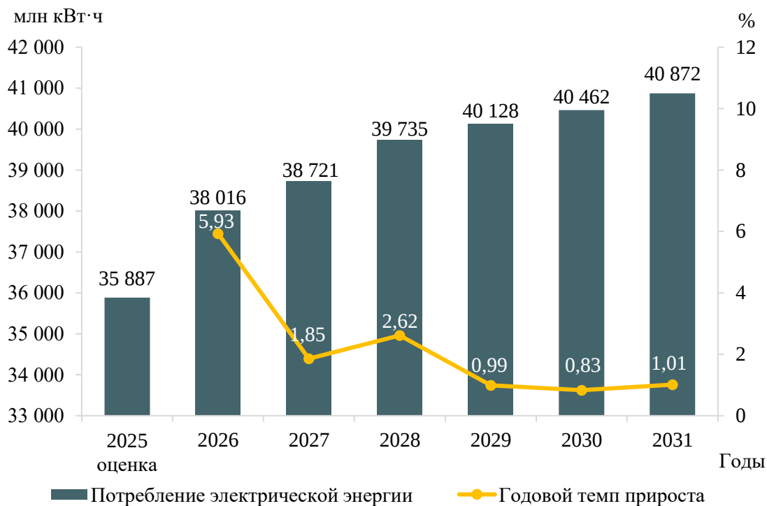
Рисунок 5 – Прогноз потребления электрической энергии энергосистемы Республики Татарстан и годовые темпы прироста
