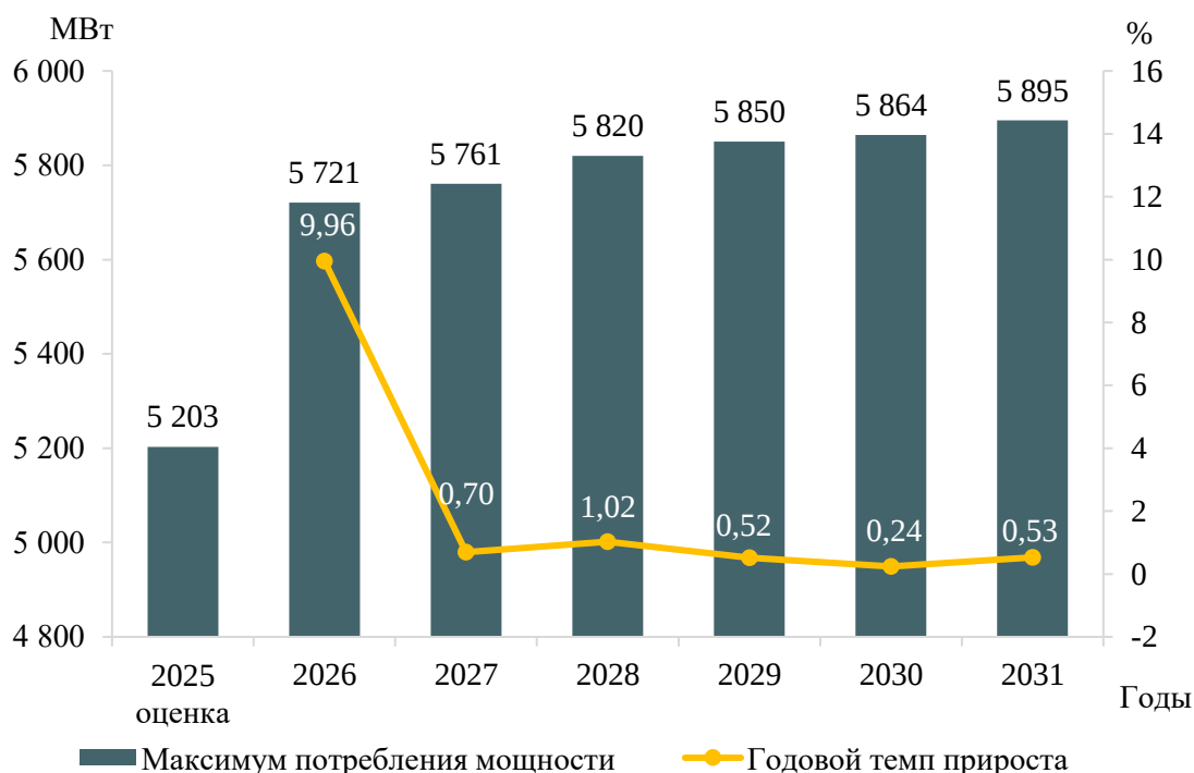
Рисунок 6 – Прогноз максимума потребления мощности энергосистемы Республики Татарстан и годовые темпы прироста
