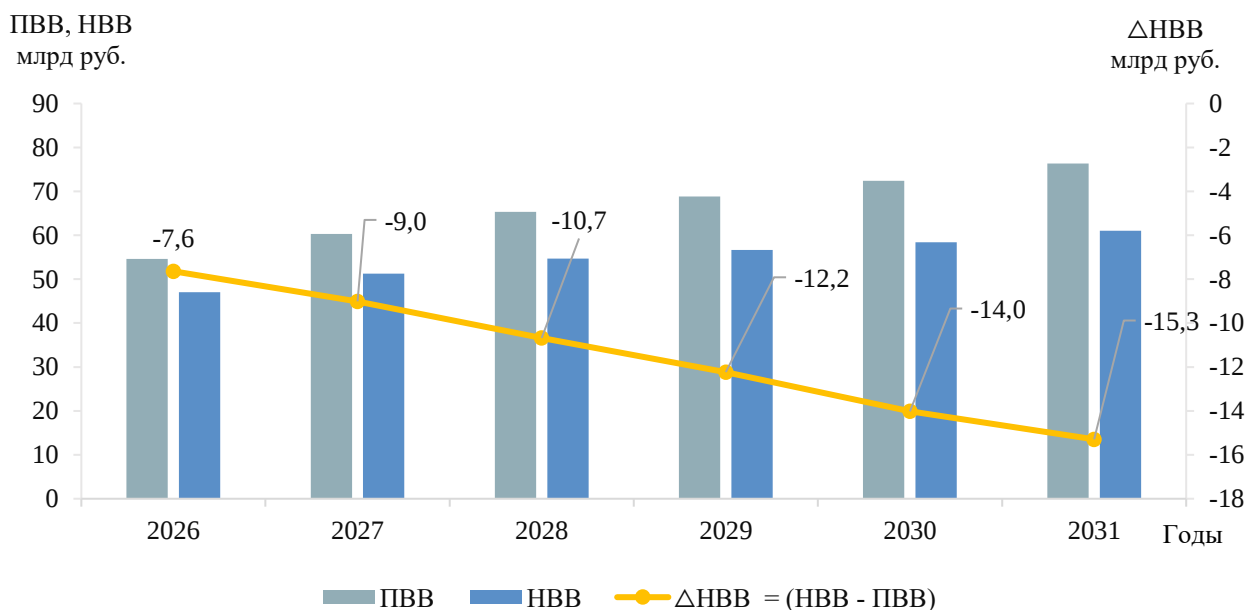
Рисунок 8 – Результаты оценки достаточности выручки, получаемой ТСО Республики Татарстан при существующих механизмах тарифного регулирования, для реализации планируемого состава технических решений, предлагаемых к включению в схему и программу развития электроэнергетических систем России (Базовый сценарий)
