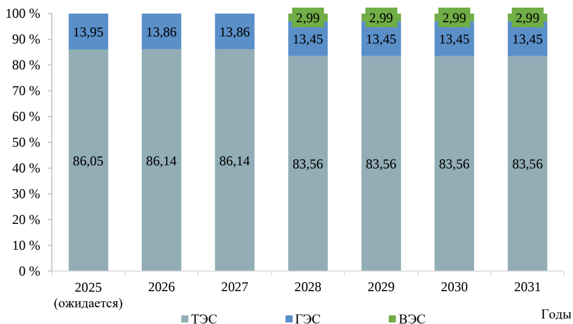
Рисунок 7 – Структура установленной мощности электростанций энергосистемы Республики Татарстан
