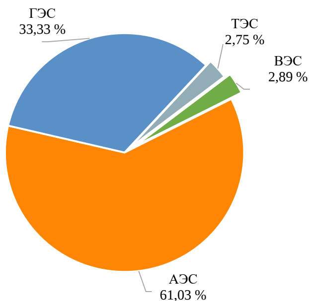
Рисунок 2 – Структура производства электрической энергии электростанций энергосистемы Мурманской области в 2024 году
