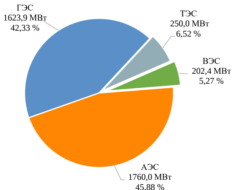
Рисунок 1 – Структура установленной мощности электростанций энергосистемы Мурманской области по состоянию на 01.01.2025
