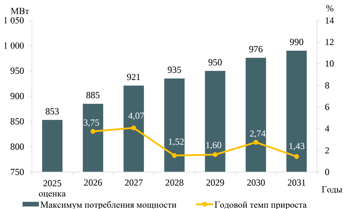
Рисунок 6 – Прогноз максимума потребления мощности и годовые темпы прироста энергосистемы Калининградской области
