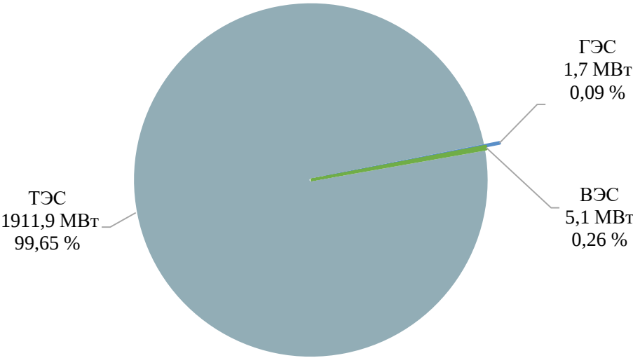
Рисунок 1 – Структура установленной мощности электростанций энергосистемы Калининградской области по состоянию на 01.01.2025
