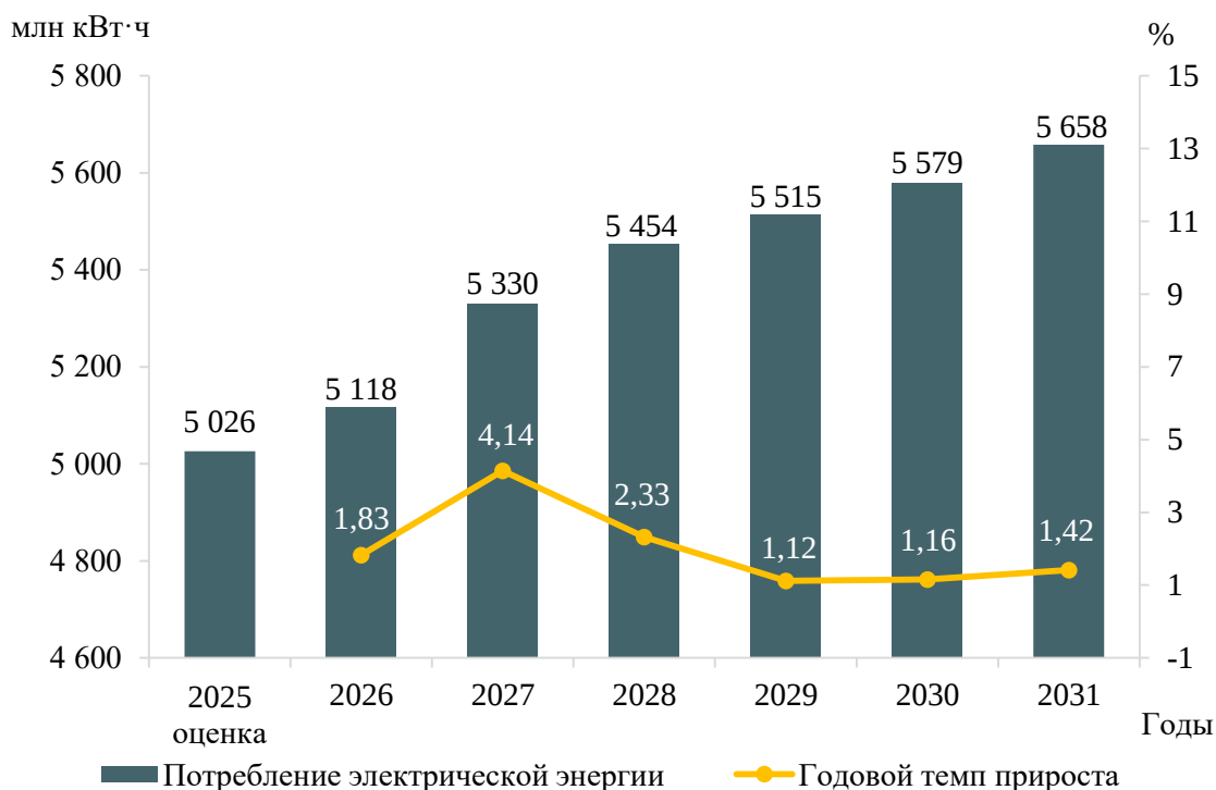
Рисунок 5 – Прогноз потребления электрической энергии энергосистемы Калининградской области и годовые темпы прироста
