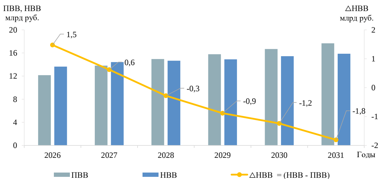
Рисунок 8 – Результаты оценки достаточности выручки, получаемой ТСО Калининградской области при существующих механизмах тарифного регулирования, для реализации планируемого состава технических решений, предлагаемых к включению в схему и программу развития электроэнергетических систем России (Базовый сценарий)
