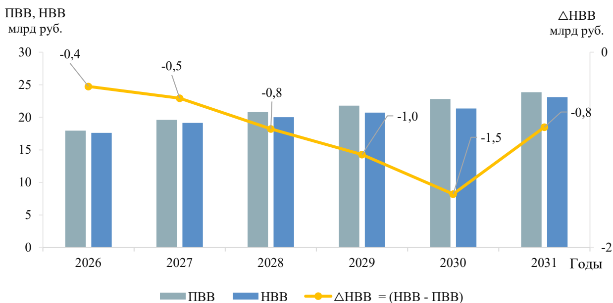
Рисунок 6 – Результаты оценки достаточности выручки, получаемой ТСО Владимирской области при существующих механизмах тарифного регулирования, для реализации планируемого состава технических решений, предлагаемых к включению в схему и программу развития электроэнергетических систем России (Базовый сценарий)
