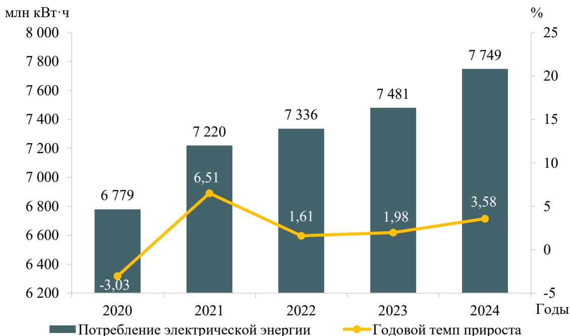
Рисунок 1 – Потребление электрической энергии энергосистемы Владимирской области и годовые темпы прироста
