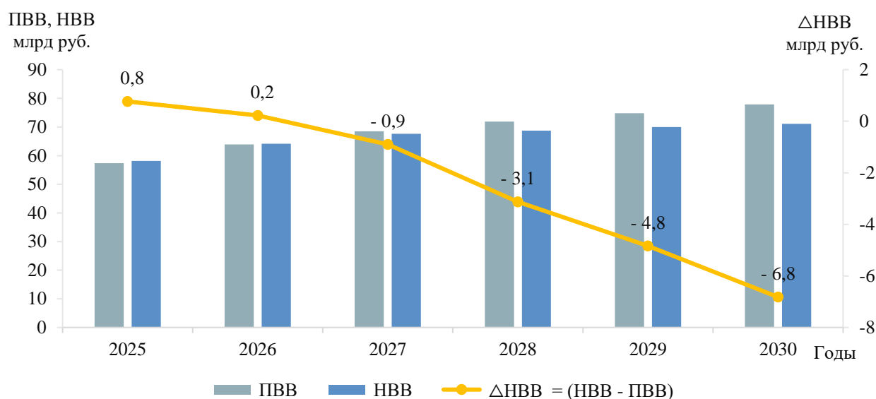
Рисунок 8 – Результаты оценки достаточности выручки, получаемой ТСО Свердловской области при существующих механизмах тарифного регулирования, для реализации планируемого состава технических решений, предлагаемых к включению в схему и программу развития электроэнергетических систем России (Базовый сценарий)
