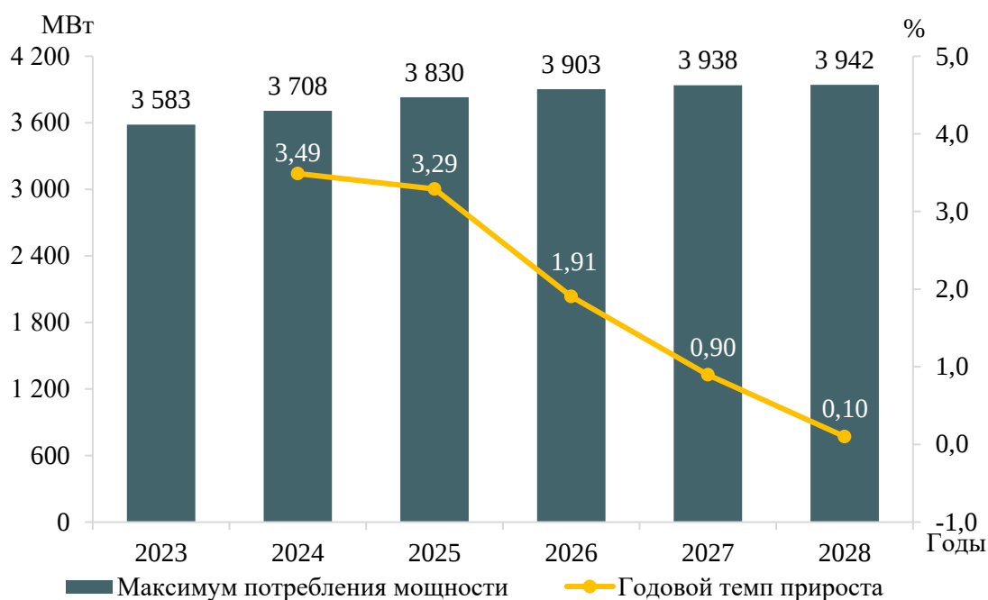
Рисунок 5 – Прогноз максимума потребления мощности энергосистемы Самарской области и годовые темпы прироста на период 2023–2028 годов
