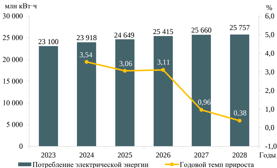
Рисунок 4 – Прогноз потребления электрической энергии энергосистемы Самарской области и годовые темпы прироста на период 2023–2028 годов
