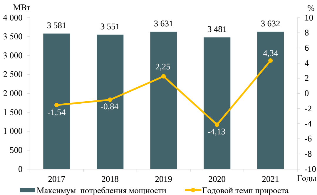
Рисунок 3 – Максимум потребления мощности энергосистемы Самарской области и годовые темпы прироста за период 2017–2021 годов
