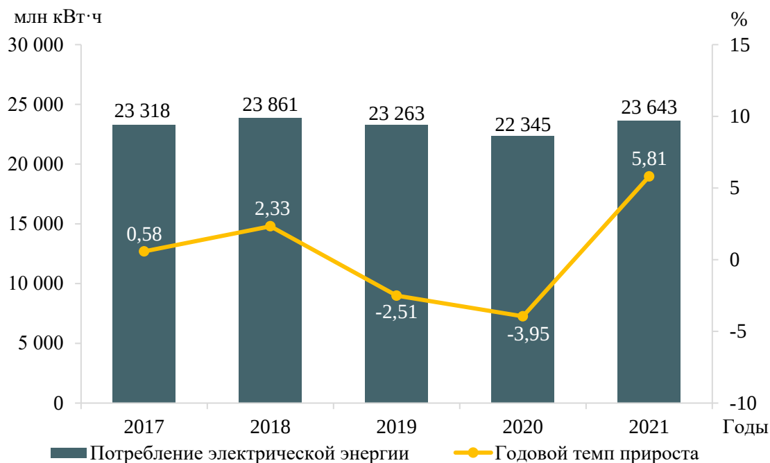
Рисунок 2 – Потребление электрической энергии энергосистемы Самарской области и годовые темпы прироста за период 2017–2021 годов
