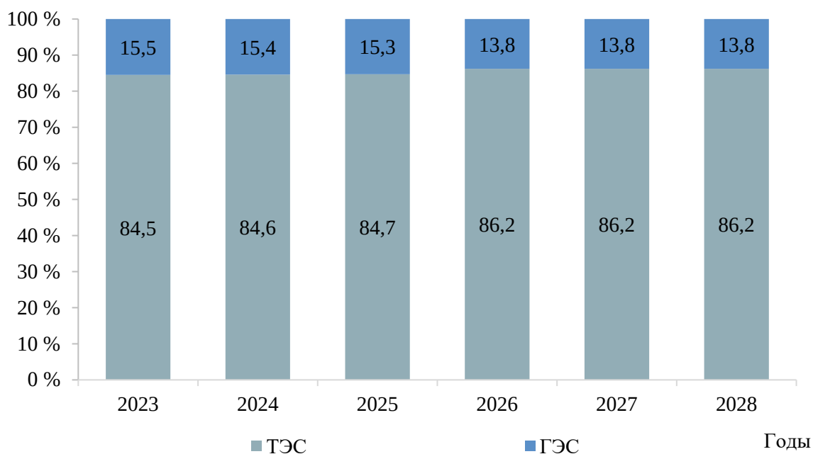
Рисунок 6 – Структура установленной мощности электростанций энергосистемы Республики Татарстан
