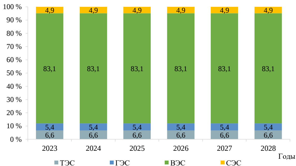
Рисунок 6 – Структура установленной мощности электростанций энергосистемы Республики Адыгея и Краснодарского края, расположенных на территории Республики Адыгея
