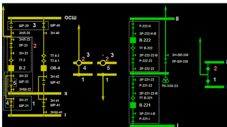
Рисунок 17. Соответствие состояний оборудования и КС
