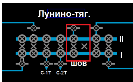
Рисунок 20. Использование КС без выключателя для шиносоединительного обходного выключателя
