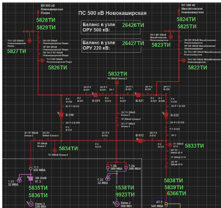
Рисунок 54. Фрагмент схемы объекта в редакторе
