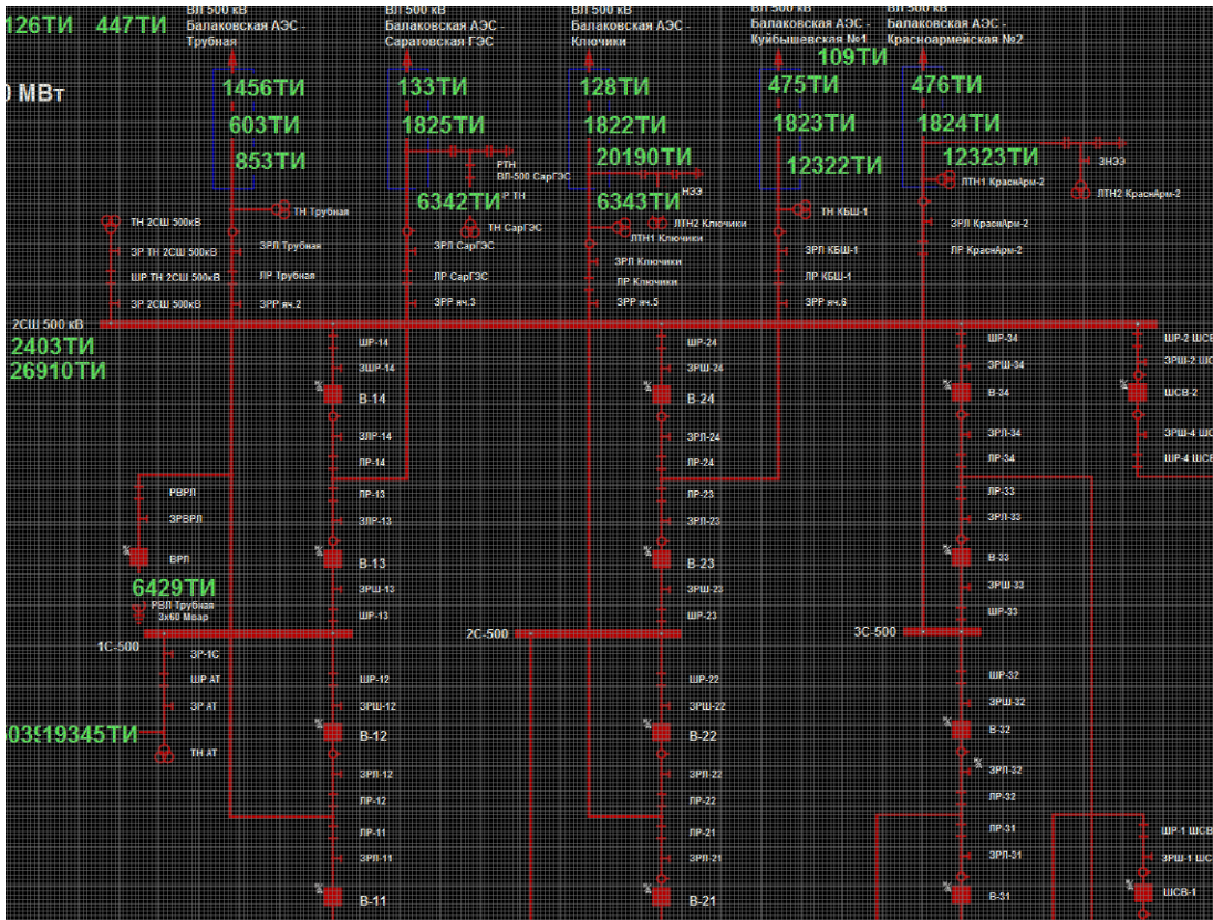
Рисунок 27. Фрагмент схемы объекта в редакторе
