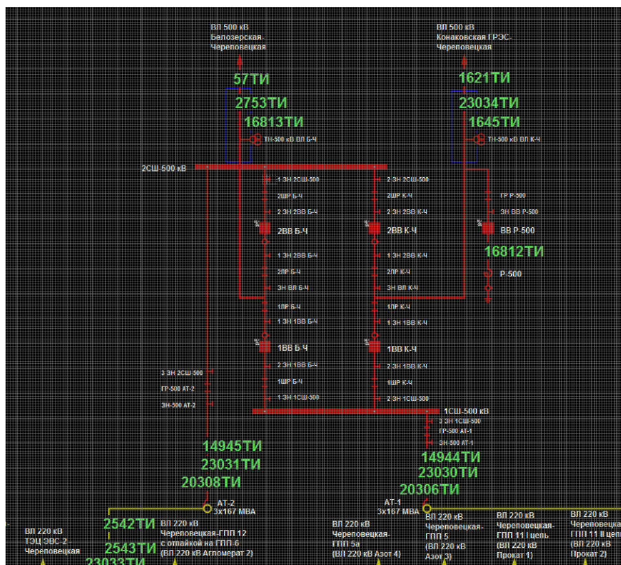
Рисунок 43. Фрагмент схемы объекта
