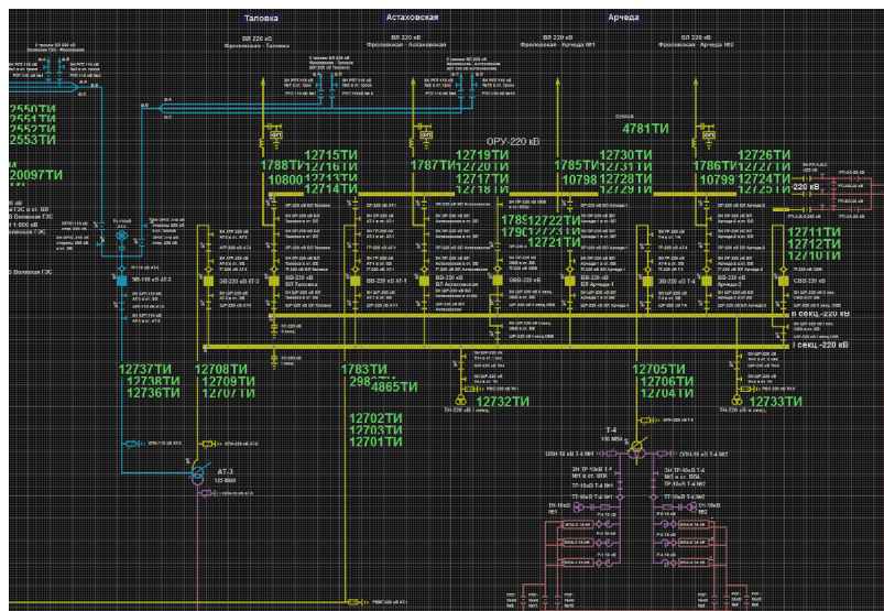
Рисунок 36. Фрагмент главной схемы
