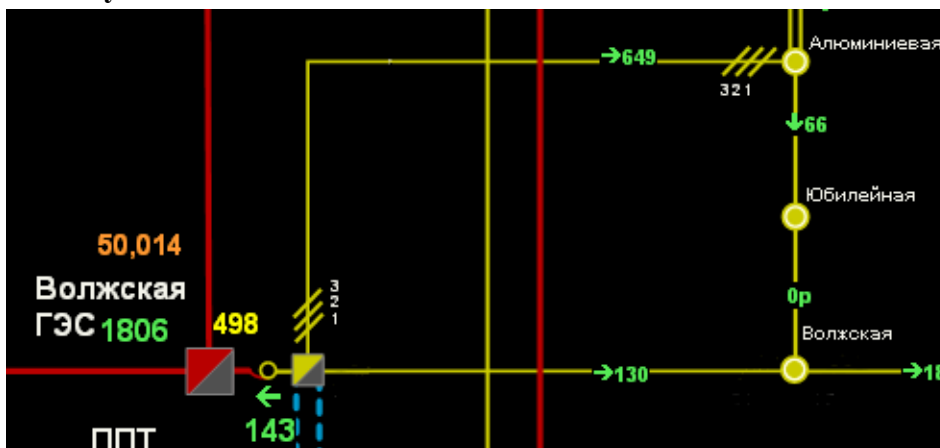
Рисунок 67. Пример режимной схемы с эквивалентной ЛЭП
