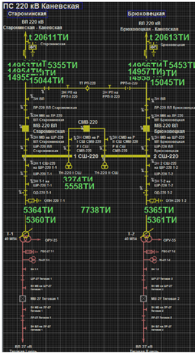
Рисунок 57. Фрагмент схемы объекта в редакторе
