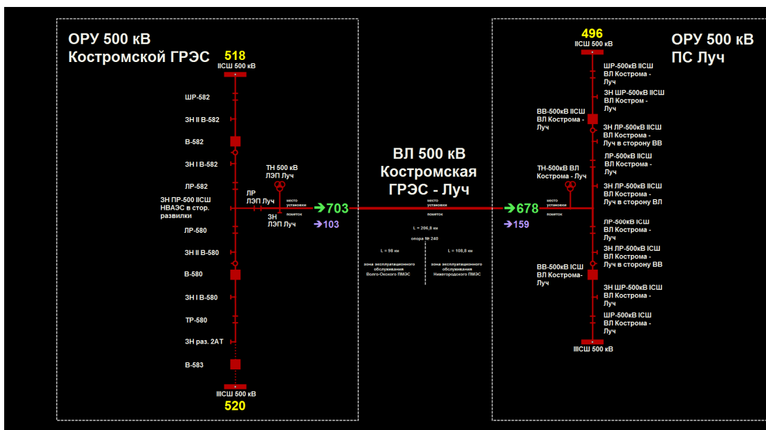
Рисунок 64. Схема ЛЭП
