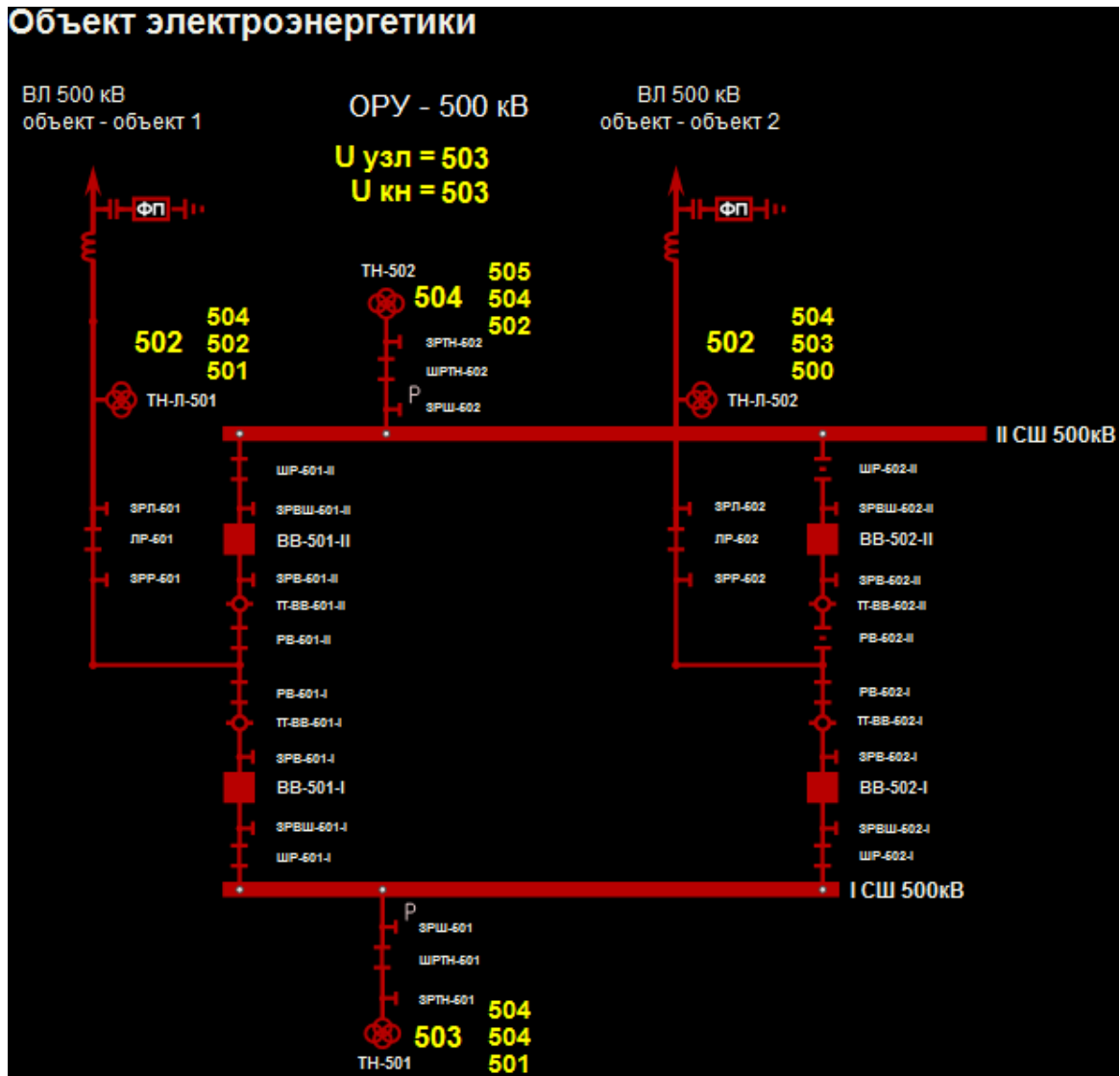
Рисунок 11. Схема ОРУ объекта (Uном=500)
