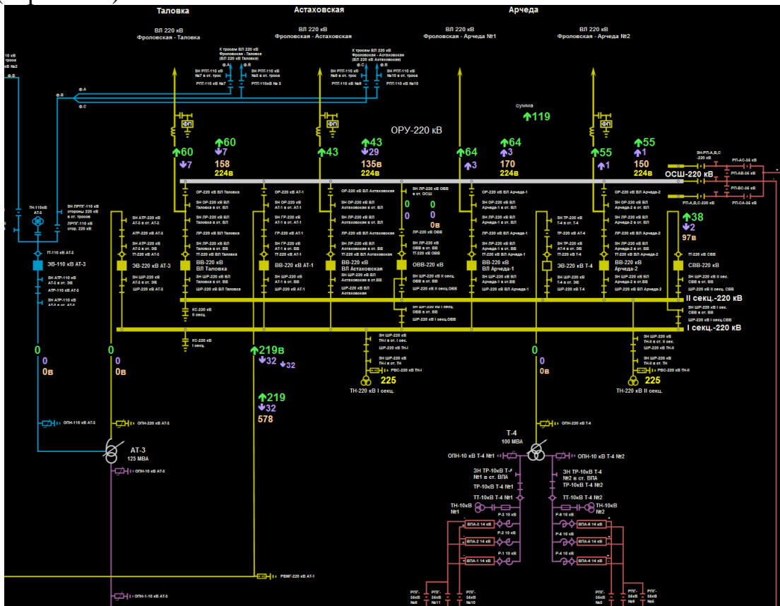
Рисунок 35. Фрагмент схемы объекта
