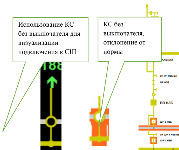
Рисунок 18. Фрагмент отображения на главной схеме и схеме объекта
