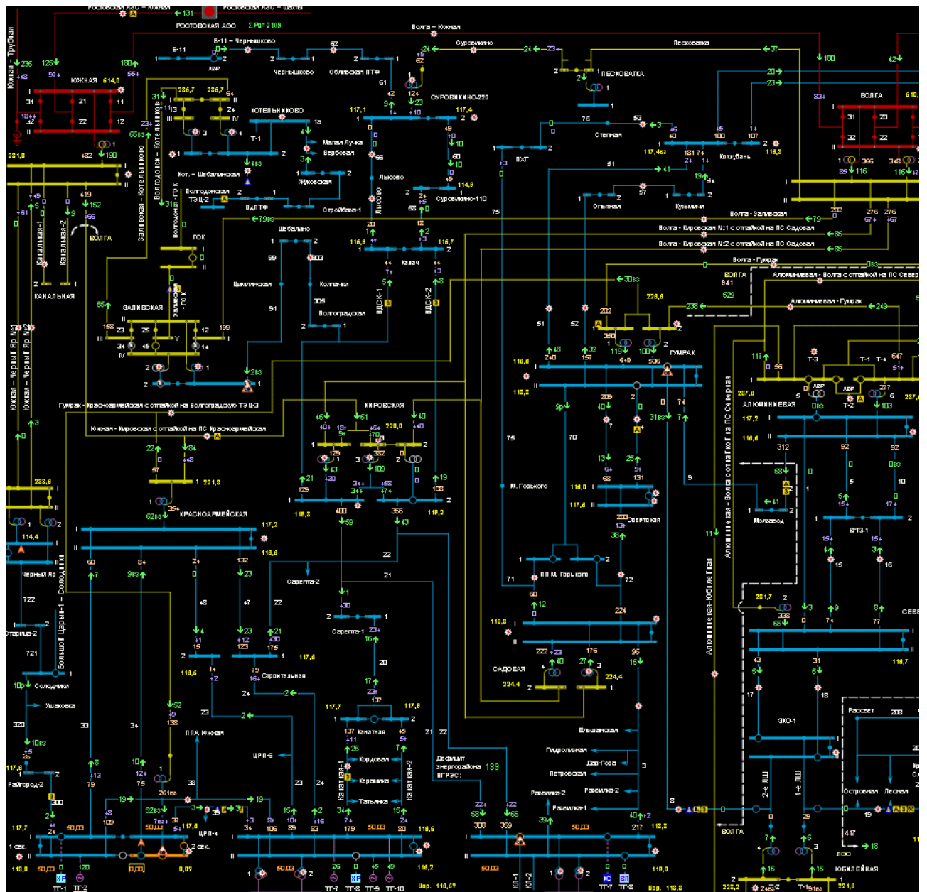
Рисунок 63. Фрагмент главной схемы
