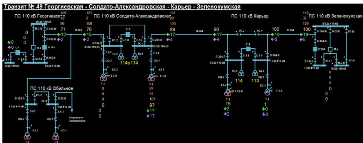
Рисунок 58. Транзит 110 кВ с отображением значений фазных токов в отключаемом слое
