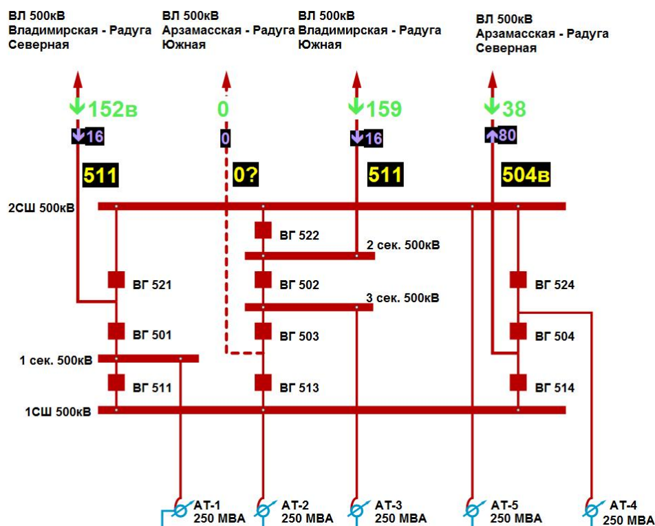
Рисунок 13. Схема объекта ПС 500 кВ Радуга
