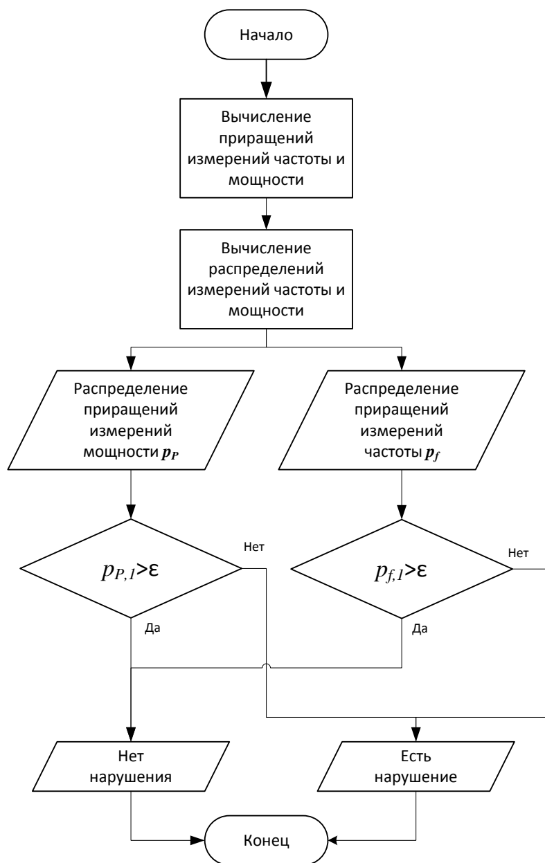
Рисунок 3. Блок-схема алгоритма "Несоответствие дискретности измерений требованиям"
